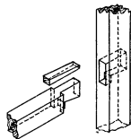
FIG. 15.—Dovetailed Tenon.
